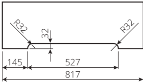
VENTILAČNÍ SEŘÍZNUTÍ LUMEN/LUMEN LOFT
