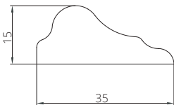
Průřez profilu dekorativní lišty
