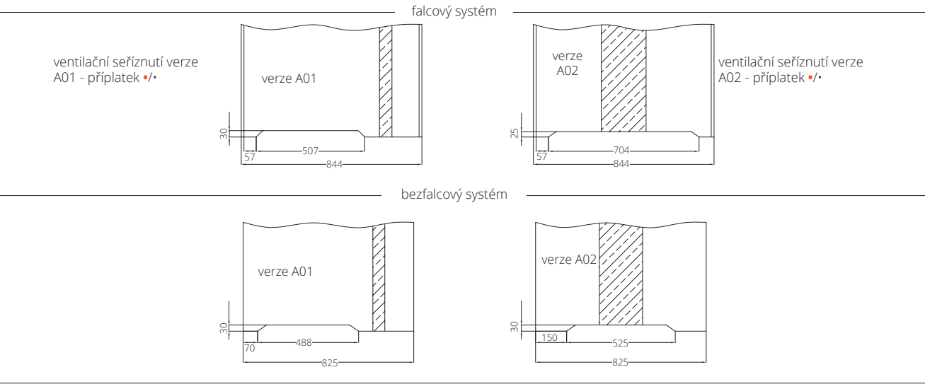
VENTILAČNÍ SEŘÍZNUTÍ LUMEN/LUMEN LOFT
