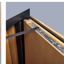
skrytý zavírač dveří
